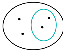
Nënbashkësi
