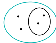
Bashkësi universale
