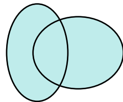
Unioni i bashkësive
