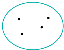
Bashkësi
