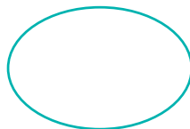
Bashkësi boshe
