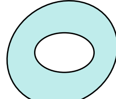
Komplementi
