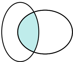
Prerja e bashkësive
