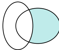
Diferenca e bashkësive
