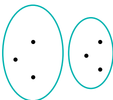
Bashkësi disjunkte
