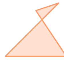
Shumëkëndësh i kryqëzuar
