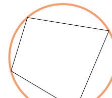
Rreth i jashtëshkruar
