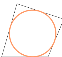
Rreth i brendashkruar
