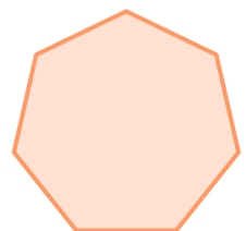
Shumëkëndësh i rregulltë
