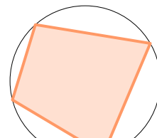
Shumëkëndësh ciklik (kordiak)
