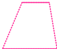
Dy baza, Dy këmbë (brinjë anësore)
