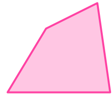
Katërkëndësh i parregullt
