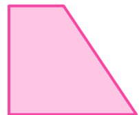
Trapez kënddrejtë
