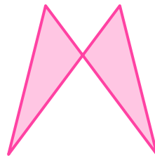
Antiparalelogramo
