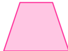
Trapezio isoszele
