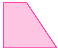
Trapezio angeluzuzen
