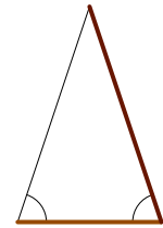
Oinarri, Alde
