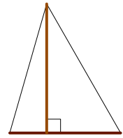
Altuera, Oinarri
