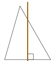
Erdibitzaile elkarzut
