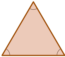
Triangelu aldekie/aldeberdin
