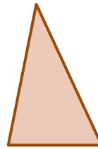
Triangelu eskaleno
