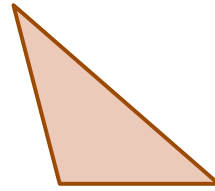
Triangelu kamuts
