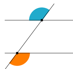
Naizmjenični vanjski uglovi
