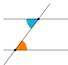
Naizmjenični unutrašnji uglovi
