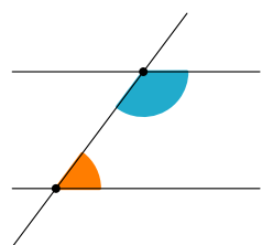
Unutrašnji uglovi na transversali
