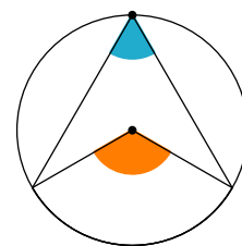
Periferijski ugao, Centralni ugao
