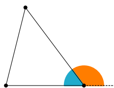
Unutrašnji ugao, Vanjski ugao
