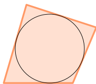
Tangentni mnogougao [primjerice tangentni četverougao]
