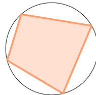
Tetivni mnogougao [primjerice tetivni četverougao]
