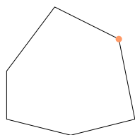
Vrh mnogougla (vrh poligona)
