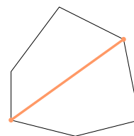
Dijagonala
