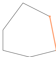
Stranica
