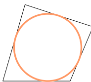
Kružnica upisana mnogouglu [primjerice četverouglu]
