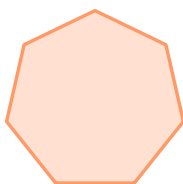
Pravilni mnogougao
