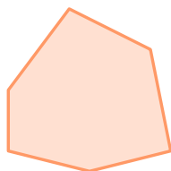
Konveksan mnogougao (konveksan poligon)
