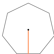
"Normala na stranicu pravilnog mnogougla"
