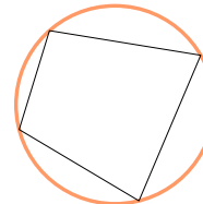
Kružnica opisana mnogouglu [primjerice četverouglu]
