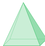
Piramida
