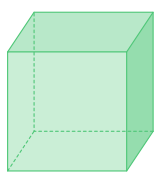
Kocka
