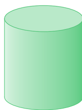
Valjak (cilindar)
