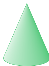
Kupa (konus)
