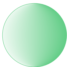
Lopta (sfera)
