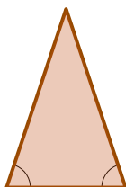
Jednakokraki trougao
