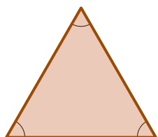
Jednakostranični trougao
