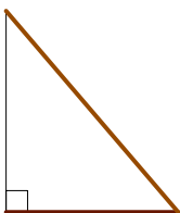
Hipotenuza, Krak
