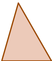
Oštrogli trougao
