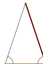
Osnovica, Krak
