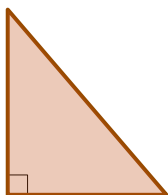
Pravougli trougao
