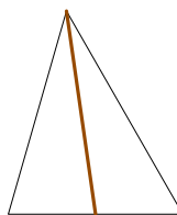
Težišnica
