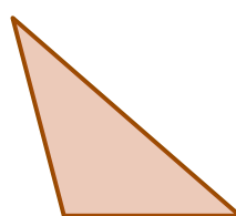
Tupougli trougao
