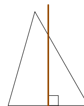
Simetrala stranice
