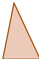
Raznostranični trougao
