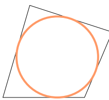
Ingeschreven cirkel
