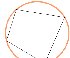
Omgeschreven veelhoek
