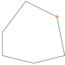
Hoekpunt
