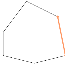
Zijde
