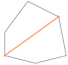
Diagonaal
