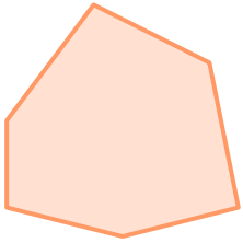
Convexe veelhoek
