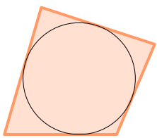
Raaklijnenveelhoek
