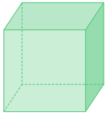
Kubus
