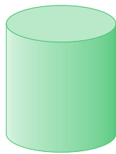
Cilinder
