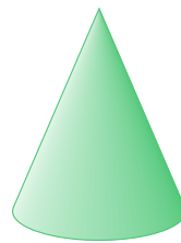
Kegel
