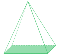
Grondvlak
