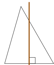
Middelloodlijn
