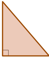
Rechthoekige driehoek
