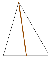
Zwaartelijn
