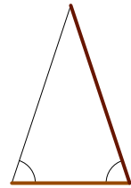
Basis, Zijde
