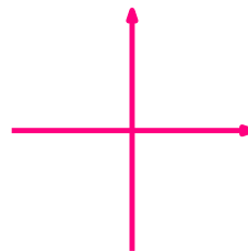
Koordinaattiakselit
