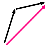
Summa (Yhteenlasku)
