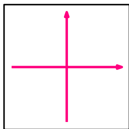
Koordinaatisto
