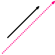
Suunta
