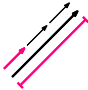
Yksikkövektori, Suuruus
