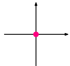
Origo
