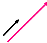
Skalaarikertolasku, Monikerta
