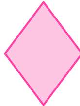
Neljäkäs
