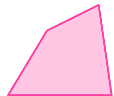
Epäsäännöllinen nelikulmio
