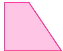
Suorakulmainen puolisuunnikas
