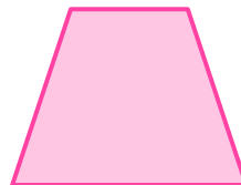
Tasakylkinen puolisuunnikas
