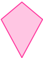
Leija
