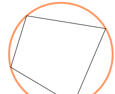
Cercle circonscrit
