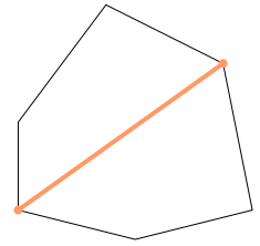
Diagonale
