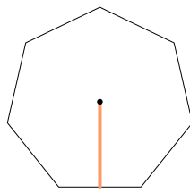
Apothème
