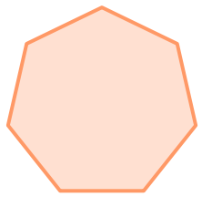
Polygone régulier
