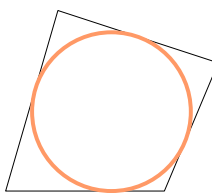
Cercle inscrit
