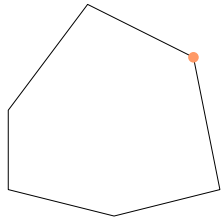
Sommet
