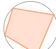
Polygone inscritible
