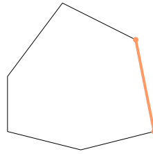
Côté
