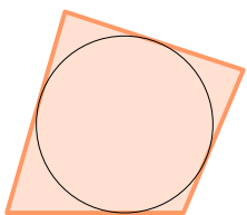
Polygone circonscriptible
