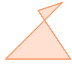
Polygone croisé
