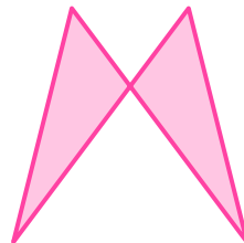
Antiparallélogramme
