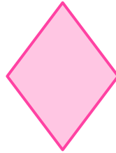
Losange
