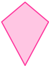
Cerf-volant convexe
