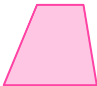
Trapèze
