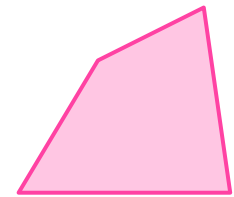
Quadrilatère irrégulier
