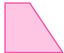
Trapèze rectangle
