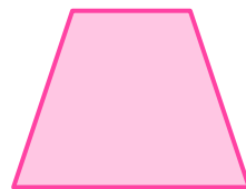
Trapèze isocèle
