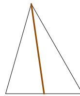
Médiane
