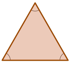
Triangle équilatéral
