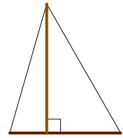
Hauteur, Base
