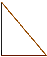
Hypoténuse, Cathète
