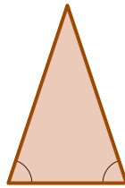
Triangle isocèle
