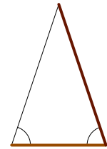
Base, Côté
