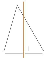
Médiatrice
