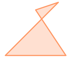
überschlagenes Polygon
