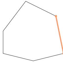
die Seite
