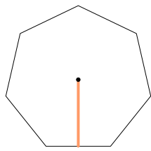
das Apothema
