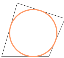
der Inkreis
