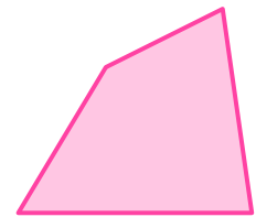
unregelmäßiges Viereck
