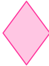
die Raute
