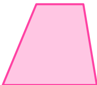
das Trapez
