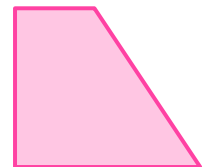
rechtwinkliges Trapez
