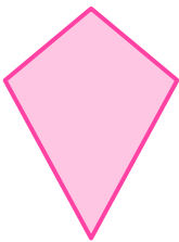
das Drachenviereck
