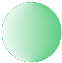
die Kugel
