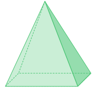
die Pyramide
