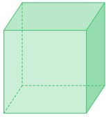
der Würfel
