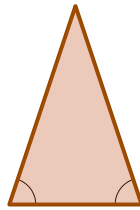
gleichschenkliges Dreieck
