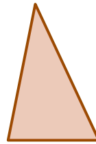
unregelmäßiges Dreieck
