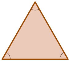
gleichseitiges Dreieck
