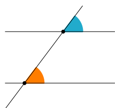
Angoli corrispondenti
