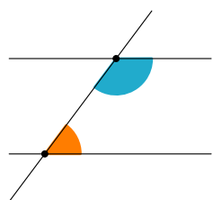
Angoli interni
