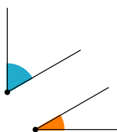
Angoli complementari
