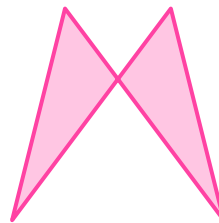
Antiparallelogramma
