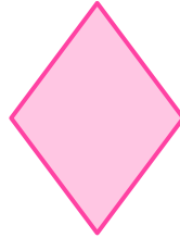
Rombo
