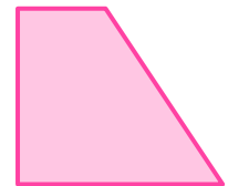
Trapezio rettangolo
