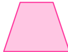
Trapezio isoscele
