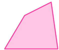
Quadrilatero irregolare
