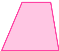
Trapezio
