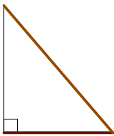
Ipotenusa, Cateto
