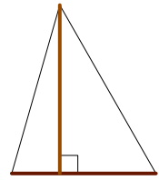
Altezza, Base
