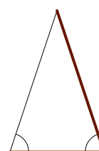
ضلع، قاعدہ
