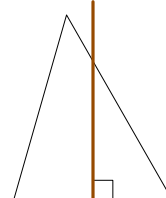
عمود منصف
