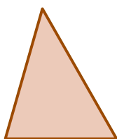
مثلث حاده
