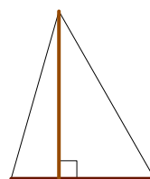
ارتفاع، قاعدہ
