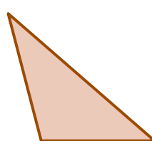
مثلث منفرجه
