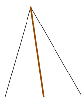
میانه
