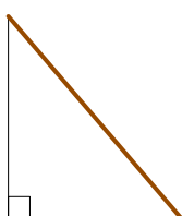
وتر، ضلع
