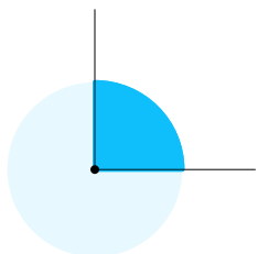
Kąt prosty
