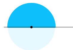
Kąt półpełny
