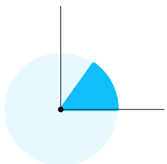
Kąt ostry
