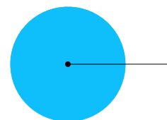
Kąt pełny
