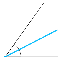
Dwusieczna
