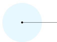
Kąt zerowy
