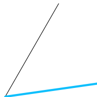
Ramię
