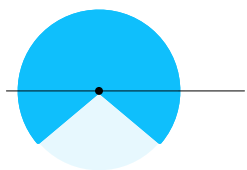
Kąt wklęsły
