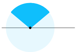
Kąt wypukły
