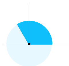
Kąt rozwarty
