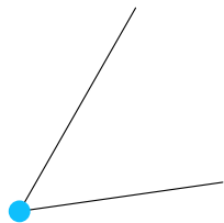
Wierzchołek
