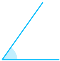
Kąt
