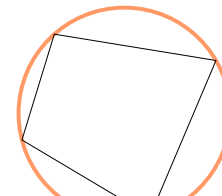
Okrąg opisany
