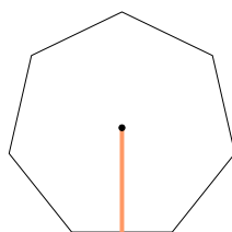
Apotema
