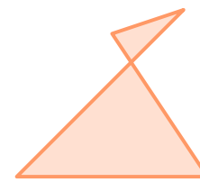
Samoprzecinający się wielokąt
