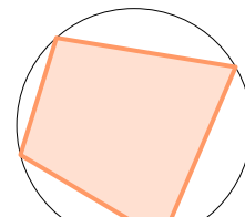
Czworokąt, na którym można opisać okrąg
