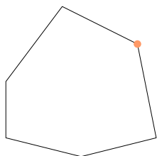
Wierzchołek
