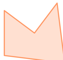
Wielokąt wklęsły
