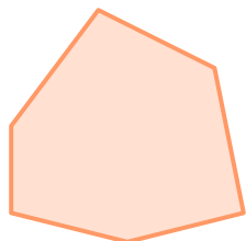
Wielokąt wypukły
