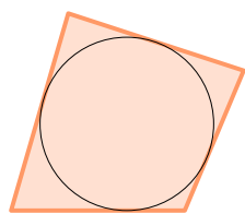
Czworokąt, w który można wpisać okrąg
