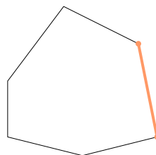
Bok
