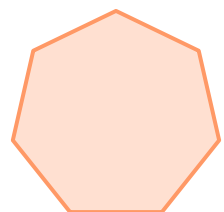
Wielokąt foremny
