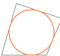
Okrąg wpisany
