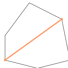
Przekątna
