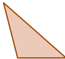
Trójkąt rozwartokątny
