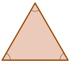
Trójkąt równoboczny
