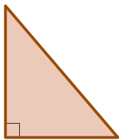
Trójkąt prostokątny
