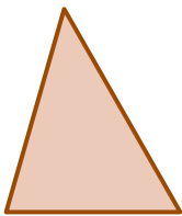
Trójkąt ostrokątny
