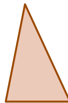
Trójkąt różnoboczny
