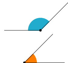
unghiuri suplementare
