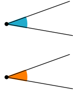
unghiuri congruente
