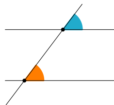
unghiuri corespondente
