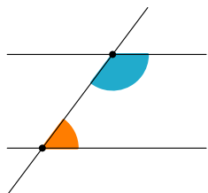
unghiuri interioare
