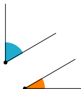
unghiuri complementare
