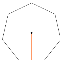
Апофема
