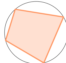
Циклический многоугольник
