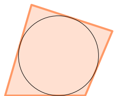
Тангенциальный многоугольник
