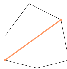
Диагональ
