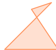
Самопересекающийся многоугольник
