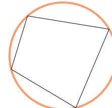
Описанная окружность
