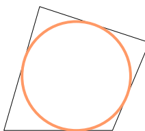
Вписанная окружность
