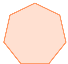
Правильный многоугольник
