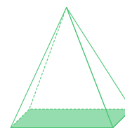
Основание пирамиды
