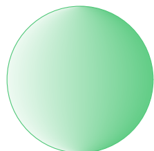
Сфера
