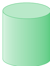
Цилиндр
