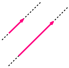
Колинеарни вектори
