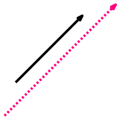
Смер
