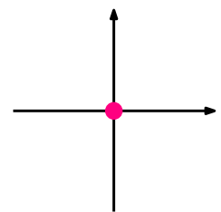
Координатни почетак
