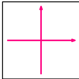
Координатни систем
