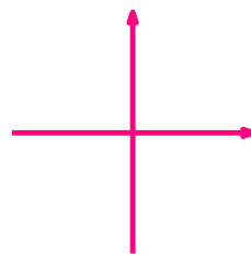
Координатне осе
