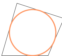
Уписана кружница
