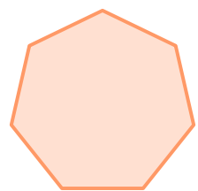
Правилан многоугао
