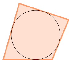
Тангентни четвороугао
