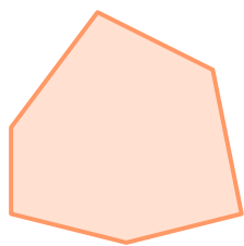
Конвексан многоугао
