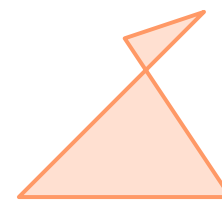
Самопресецајући многоугао
