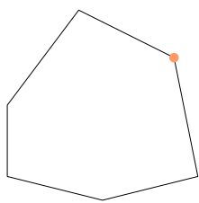
Теме многоугла
