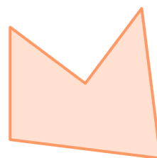
Конкавни многоугао
