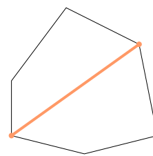
Дијагонала многоугла
