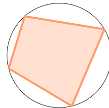
Тетивни четвороугао
