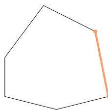
Страница многоугла
