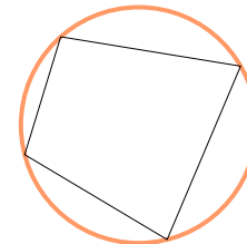
Описана кружница
