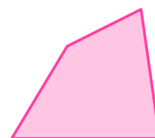
Неправилни четвороугао
