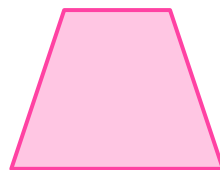
Једнакокрази трапез
