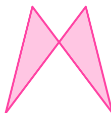
Антипаралелограм
