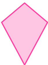
Конвексни делтоид
