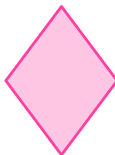
Ромб
