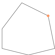
顶点
