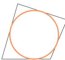
内切圆
