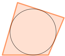
yuán wài qiē duō biān xíng
