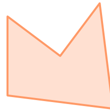
āo duō biān xíng
