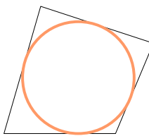
nèi qiē yuán
