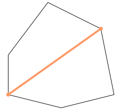
duì jiǎo xiàn
