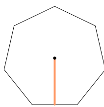
边心距
