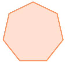
zhèng duō biān xíng
