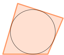
圆外切多边形
