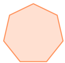
正多边形
