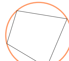
外接圆
