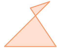
zì xiāng jiāo duō biān xíng
