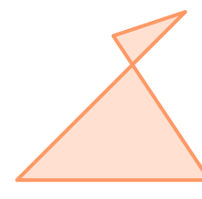
自相交多边形
