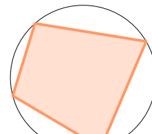
圆内接多边形
