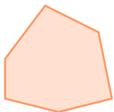
凸多边形
