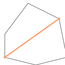
对角线
