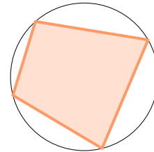
yuán nèi jiē duō biān xíng
