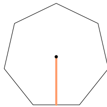
biān xīn jù
