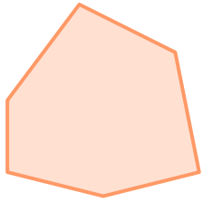
tū duō biān xíng
