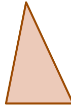
bù děng biān sān jiǎo xíng
