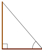
duì biān, lín biān
