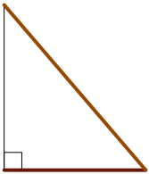
斜边 (弦) 直角边 (勾、股)
