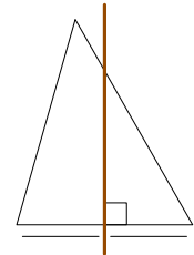
zhōng chuí xiàn (chuí zhí píng fēn xiàn)
