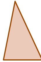
不等边三角形
