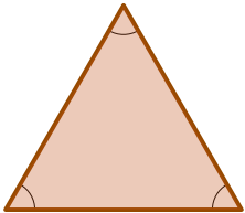
děng biān sān jiǎo xíng
