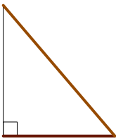
xié biān (xián), zhí jiǎo biān (gōu, gǔ)
