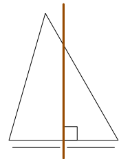
中垂线 (垂直平分线)
