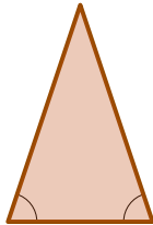
děng yāo sān jiǎo xíng
