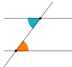
Ángulos alternos
