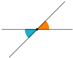
Ángulos opuestos
