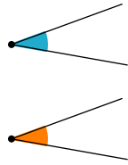
Ángulos iguales
