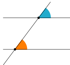
Ángulos correspondientes
