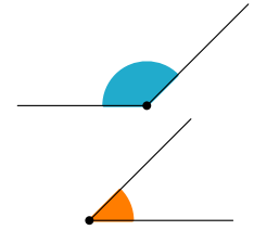
Ángulos suplementarios
