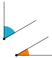
Ángulos complementarios
