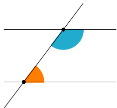
Ángulos interiores
