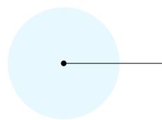
"Ángulo de 0°"
