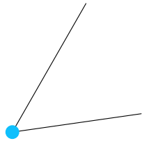
Vértice
