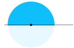
Ángulo llano
