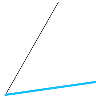
Segmento
