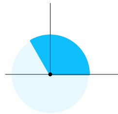
Ángulo obtuso
