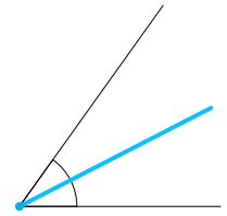
Bisectriz
