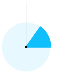
Ángulo agudo
