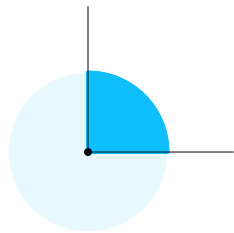
Ángulo recto
