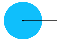
Ángulo completo
