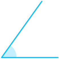
Ángulo
