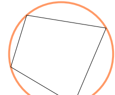
Circunferencia circunscrita
