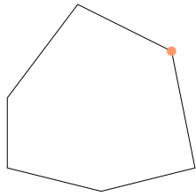
Vértice
