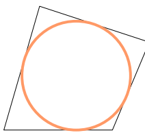
Circunferencia inscrita
