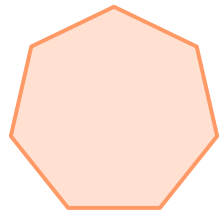
Polígono regular
