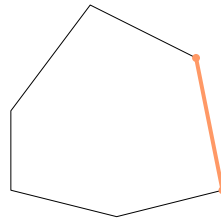
Lado
