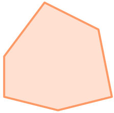
Polígono convexo
