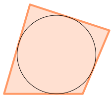
Polígono inscriptible
