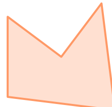
Polígono cóncavo
