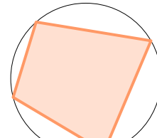
Polígono cíclico
