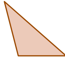
Trubbvinklig triangel
