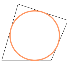
內切圓
