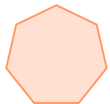
正多邊形
