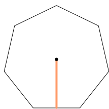
邊心距
