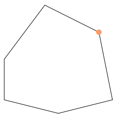
頂點
