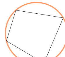
外接圓
