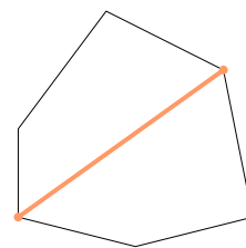
對角線
