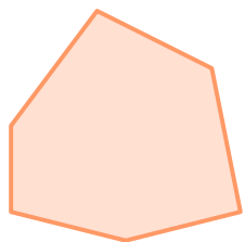
凸多邊形
