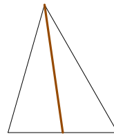
中線
