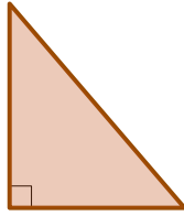
直角三角形
