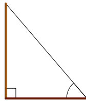
對邊，鄰邊
