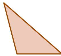
鈍角三角形
