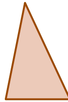
不等邊三角形
