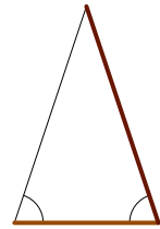
底邊，腰
