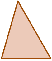
銳角三角形
