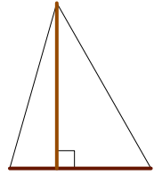
高，底
