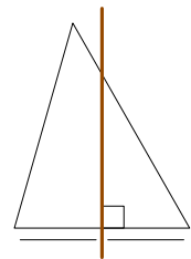
中垂線 (垂直平分線)
