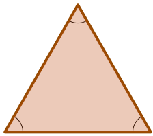
等邊三角形
