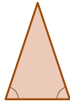
等腰三角形
