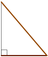
斜邊 (弦) 直角邊 (勾、股)
