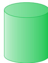
Об'єм
