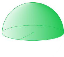
Півсфера
