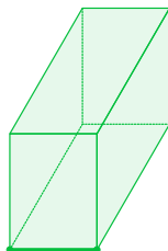
Ширина
