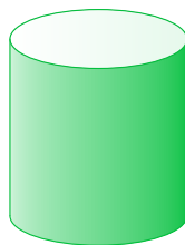
Площа
