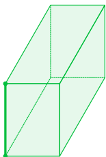
Висота
