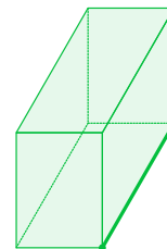
Довжина
