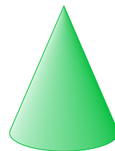
Конус
