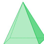
Піраміда
