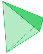
Тетраедр
