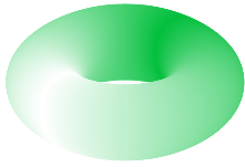
Тор
