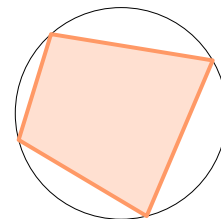
циклічний багатокутник
