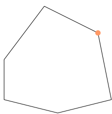
вершина
