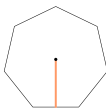
апофема
