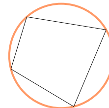
описане коло
