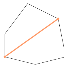
діагональ
