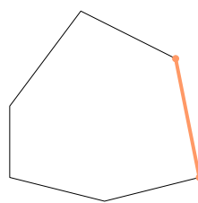
сторона
