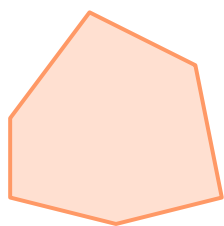
опуклий багатокутник
