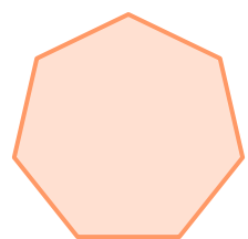
правильний багатокутник
